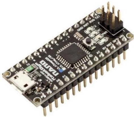
Arduino Nano v3 (Micro USB ) Compatible 328 ATmega328P
